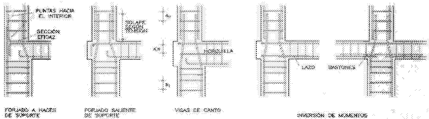
Figura 4.18. Nudos intermedios.
