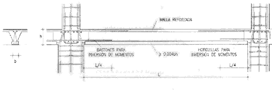
Figura 4.20. Requisitos de forjados para a_c \geq 0,16 g .
