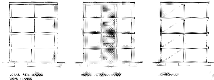
Figura 3.6.- Ejemplos de organizaciones estructurales que permiten un valor del coeficiente de comportamiento por ductilidad \mu = 2 .
