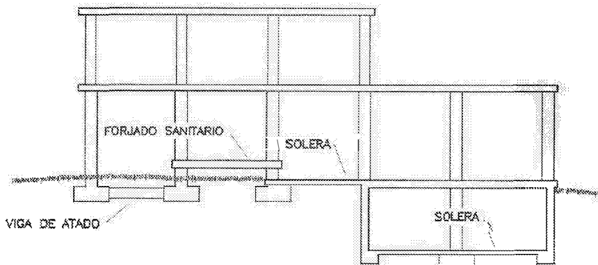
Figura 4.3. Disposición de elementos de atado.
