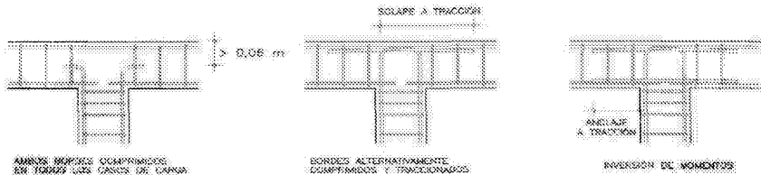
Figura 4.19. Nudos superiores.
