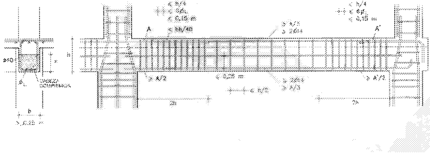
Figura 4.5. Requisitos de vigas para ductilidad muy alta ( \mu=4 ).
