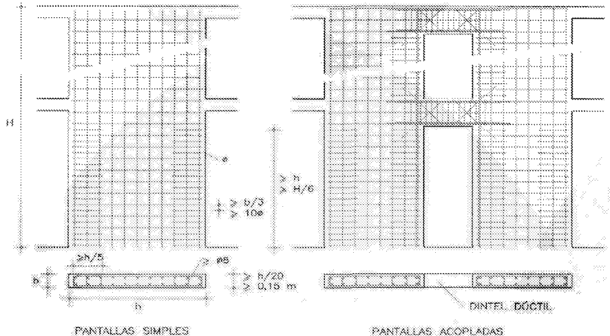
Figura 4.21. Armado de pantallas.
