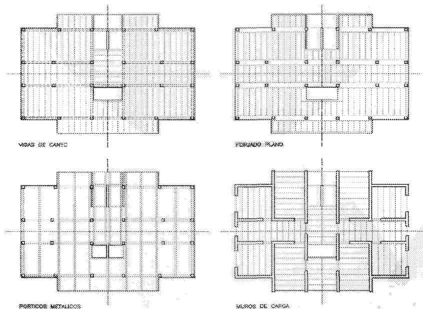
Figura 4.1. Disposiciones con simetría geométrica y mecánica.
