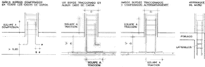
Figura 4.17. Arranque de armaduras de espera de soporte.
