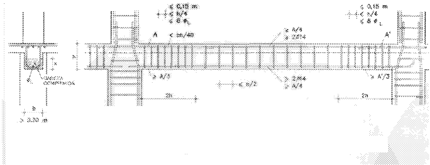
Figura 4.4. Requisitos de vigas para ductilidad alta ( \mu=3 ).
