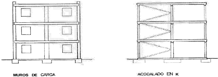
Figura 3.7.- Ejemplos de organizaciones estructurales que permiten un valor del coeficiente de comportamiento por ductilidad \mu = 1 .
