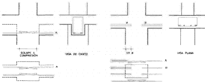
Figura 4.12. Solape de armadura inferiores.
