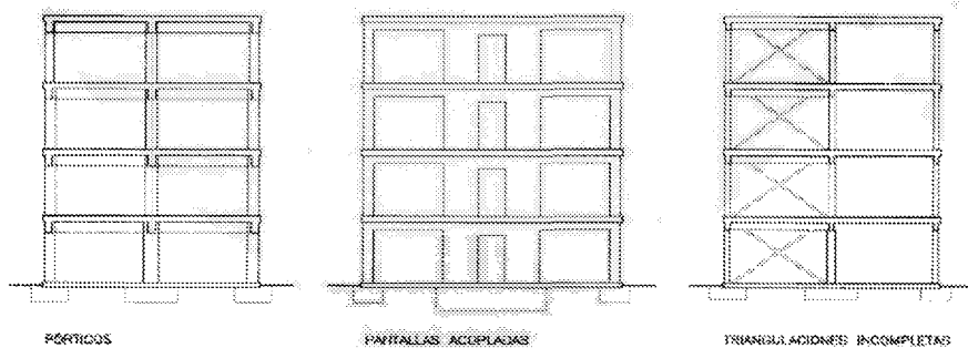
Figura 3.4.- Ejemplos de organizaciones estructurales que permiten un valor del coeficiente de comportamiento por ductilidad \mu = 4 .
