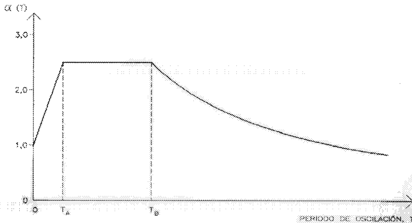
Figura 2.2. - Espectro de respuesta elástica.
