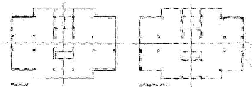
Figura 4.2. Disposiciones de elementos resistentes.
