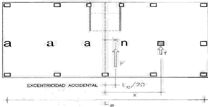
Figura 3.8. Efectos de rotación.
