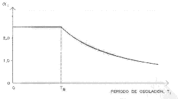
Figura 3.3. Coeficiente ar para el método simplificado de cálculo.
